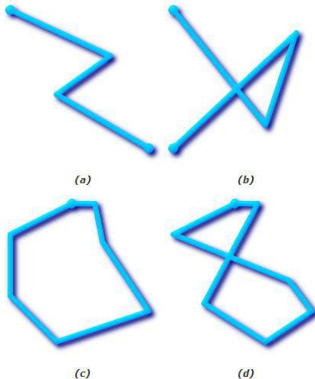
Les polygones (a) et (c) sont simples, mais pas les polygones (b) et (d)
